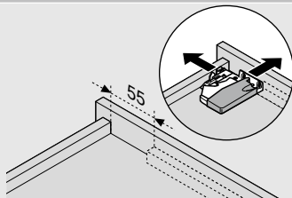
T65.1000.02 sz. fúrósablon használata
