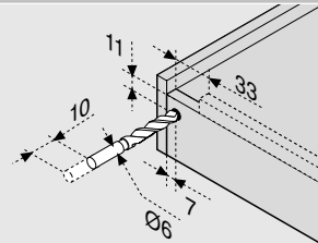
T65.1000.02 sz. fúrósablon használata
