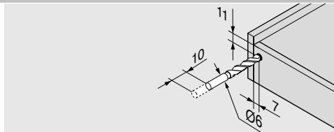
T65.1000.02 sz. fúrósablon használata
