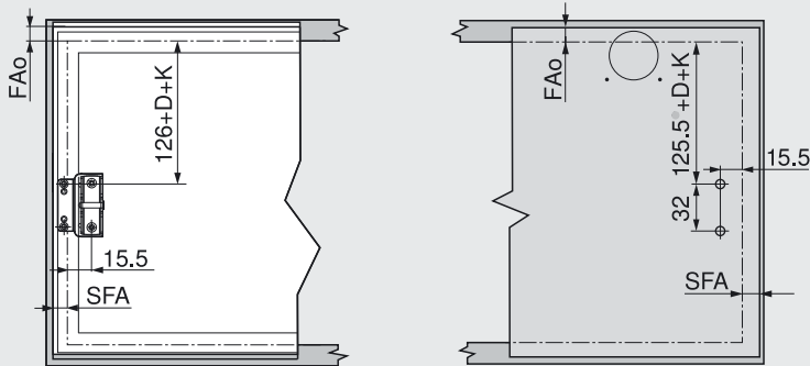
Keskeny alukeretek
